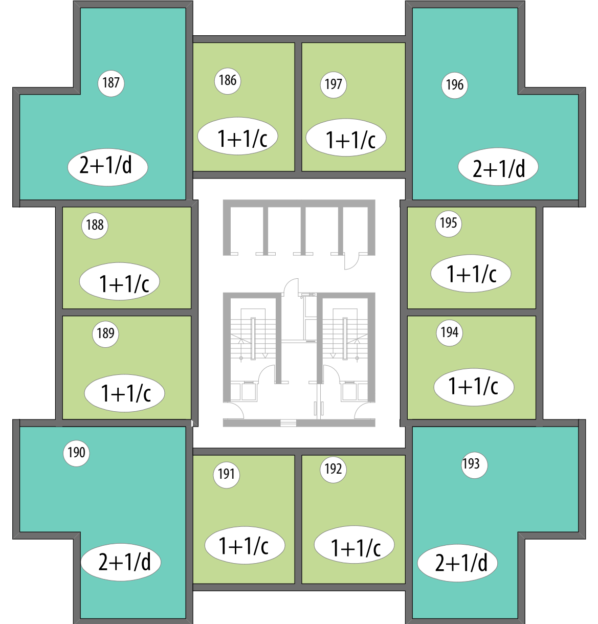
G BLOK 16.KAT PLANI
