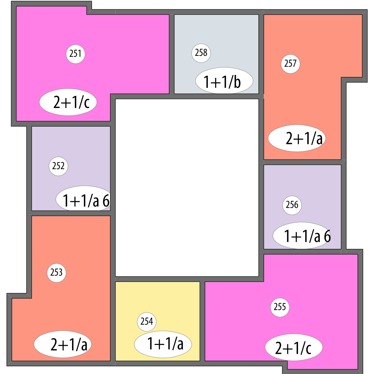
A BLOK 32.KAT PLANI
