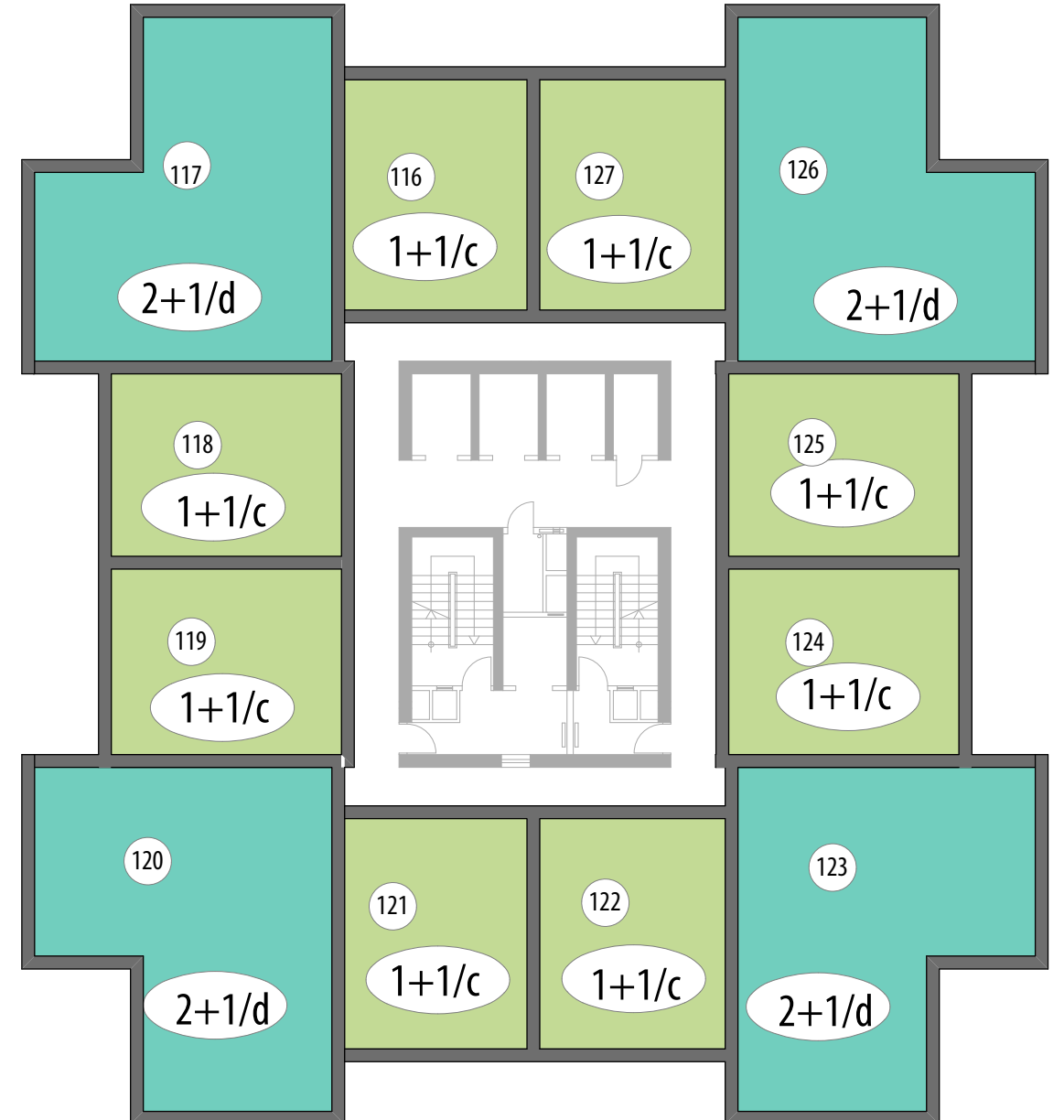
G BLOK 10.KAT PLANI
