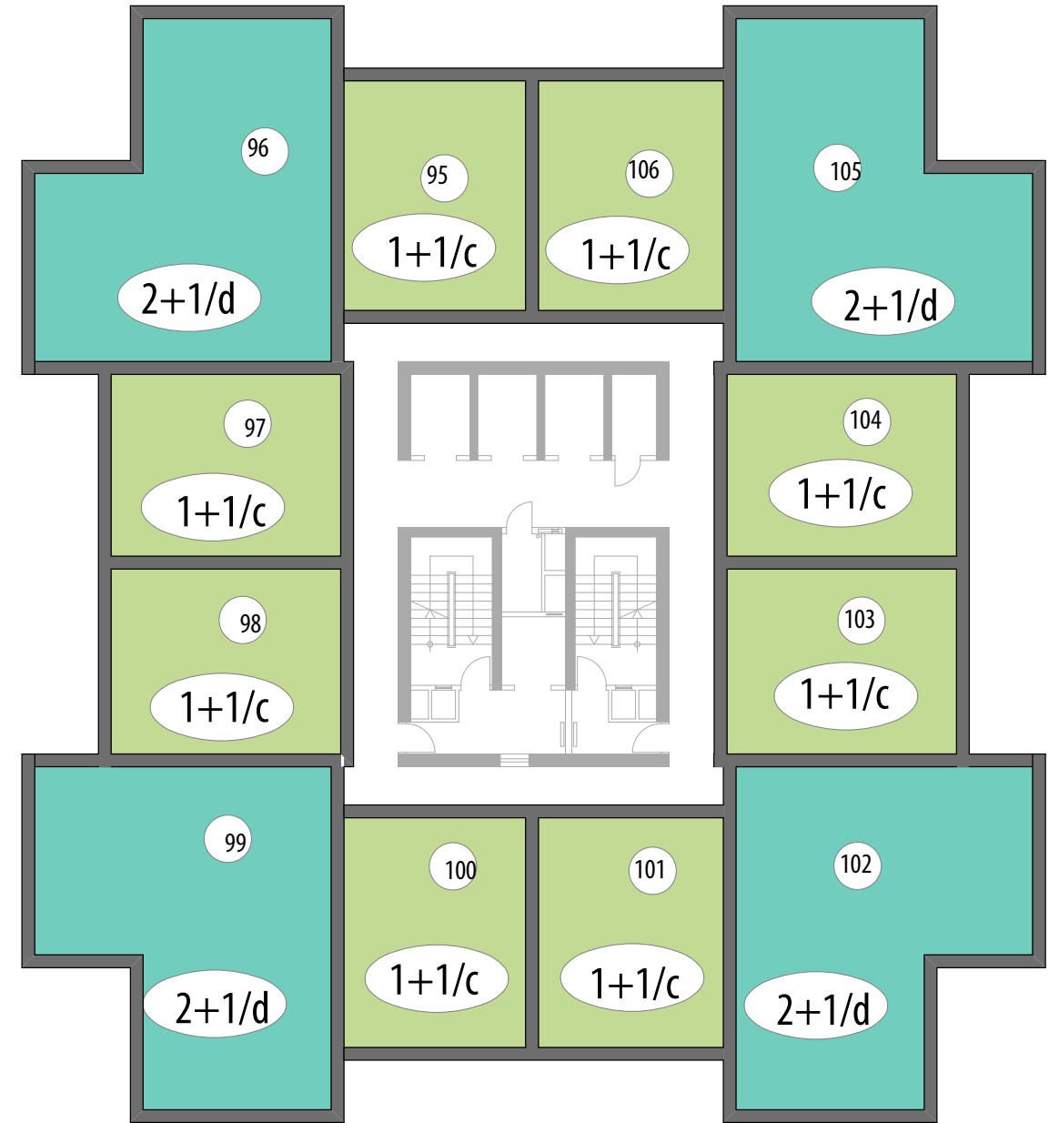
H BLOK 8.KAT PLANI
