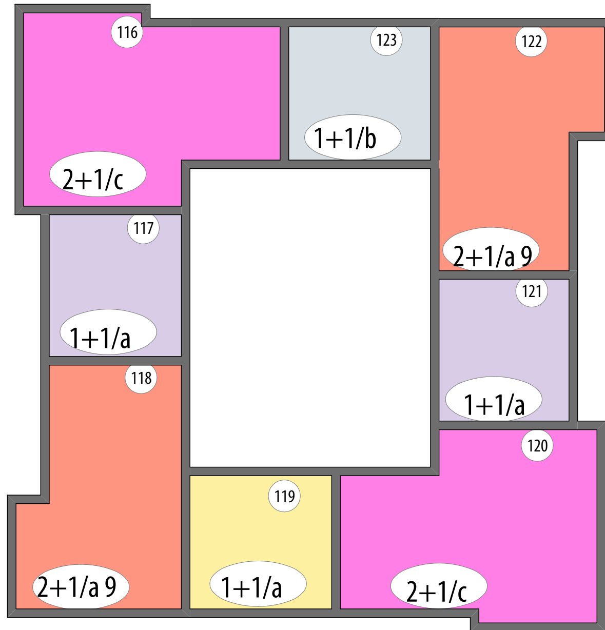
A BLOK 15.KAT PLANI
