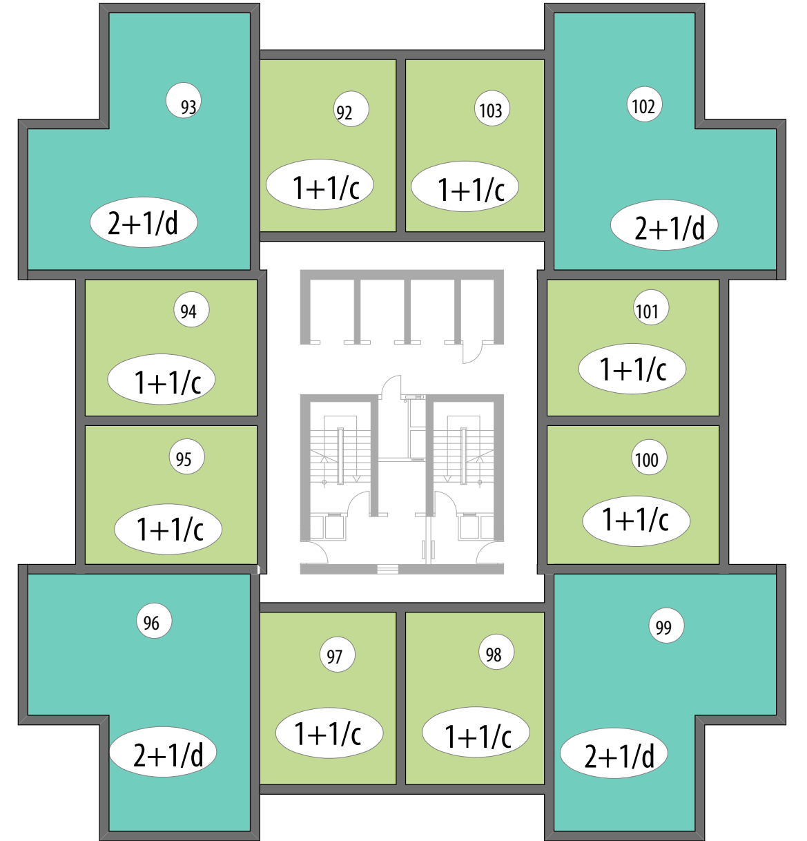
G BLOK 8.KAT PLANI
